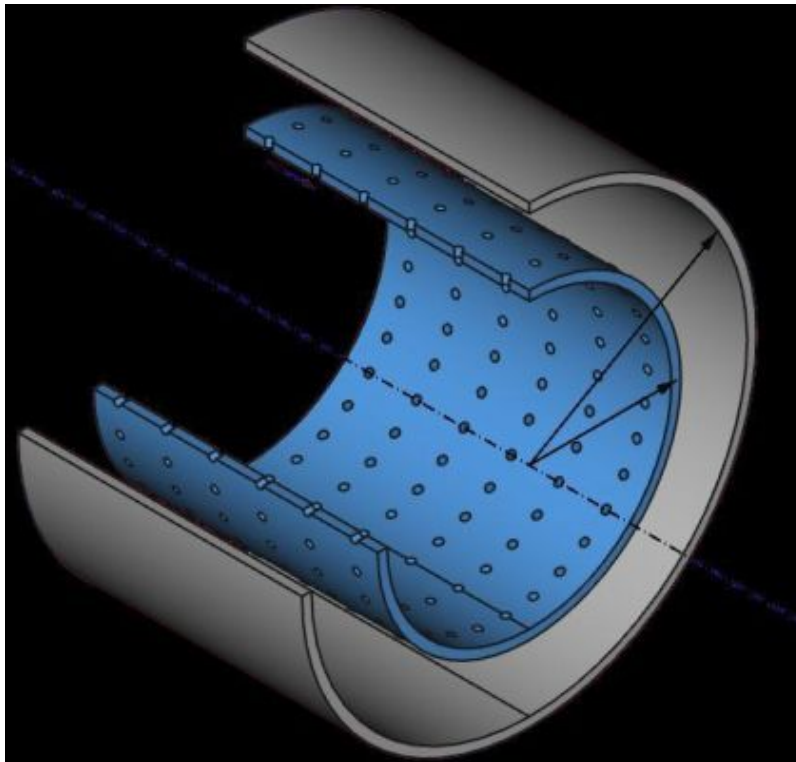
Perforierter Schallschutz für Triebwerke (Grafik: Schmidt/MATHEON)
