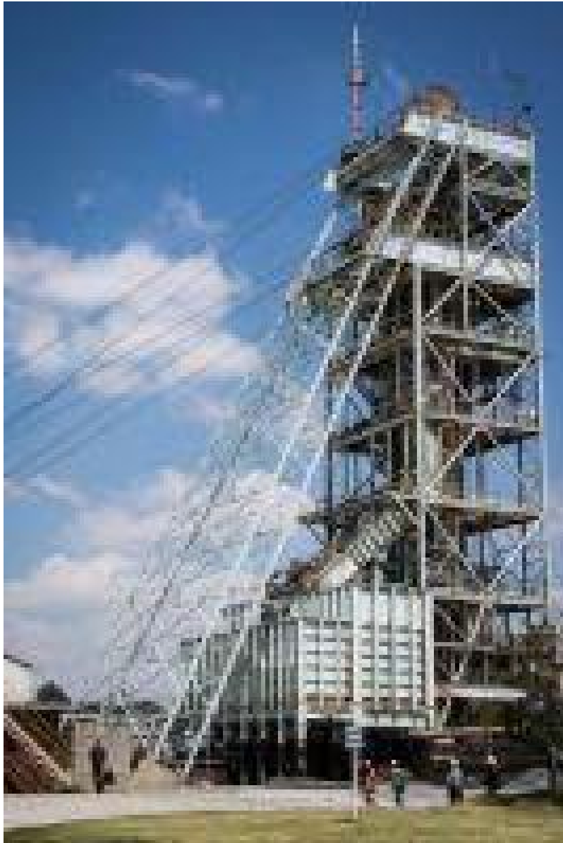
Schachtaufzug Beatrix Betrieb, Sibanye Gold, Südafrika
