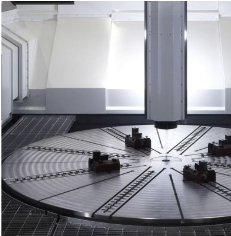
UNISIGN Dreh-Fräszentrum
