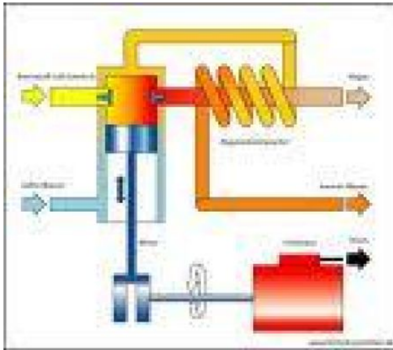
Schema BHKW
