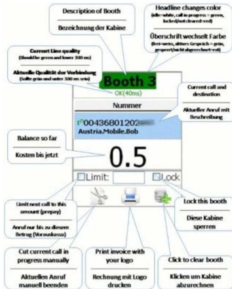
Abrechnungsschnittstelle für Callshops
