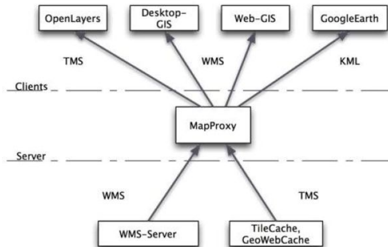
Einsatz MapProxy
