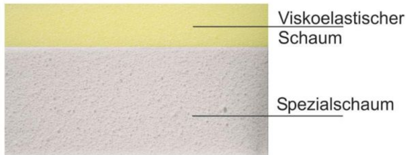
GEFATEX®-Matratze „Heavy Safe“, Aufbau der Schichten.
