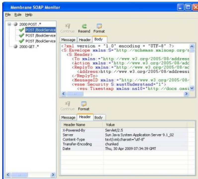
SOAP Nachricht im Monitor
