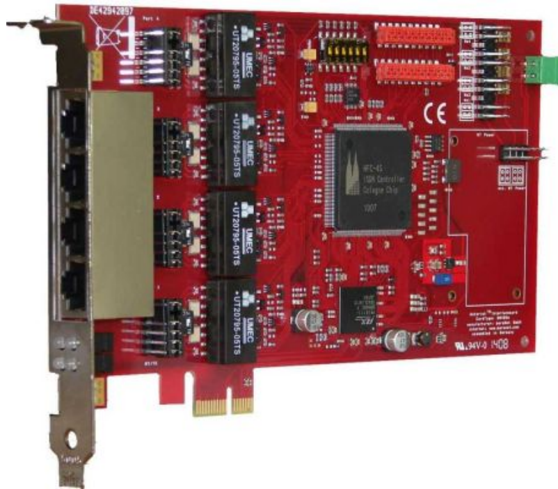
BN4S0e - PCI Express
