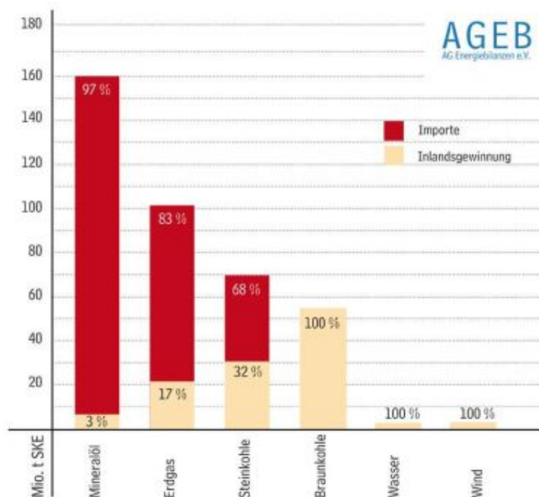
Importabhängigkeit verschiedener Energieträger in Prozent vom Gesamtverbrauch 2007
