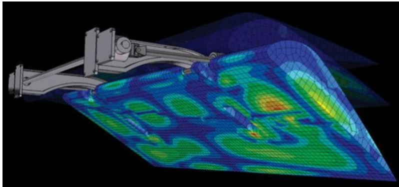
Simulation einer Landeklappe mit SimXpert
