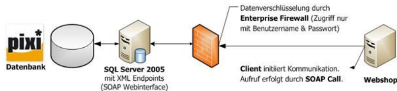
Pixi* API Architektur
