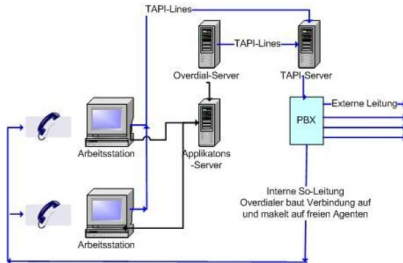
Architektur des AG-Overdial-Servers
