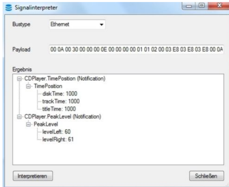
Anwendungsbeispiel zur Signal-Auswertung realisiert mit dbImporter/msgInterpreter
