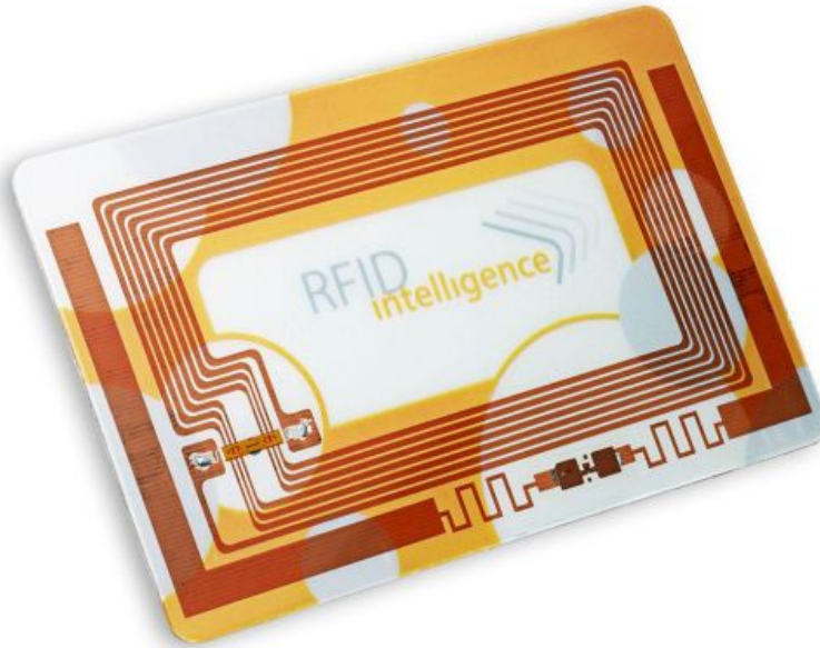
UHF Karte mit bis zu 5m Lesereichweite
